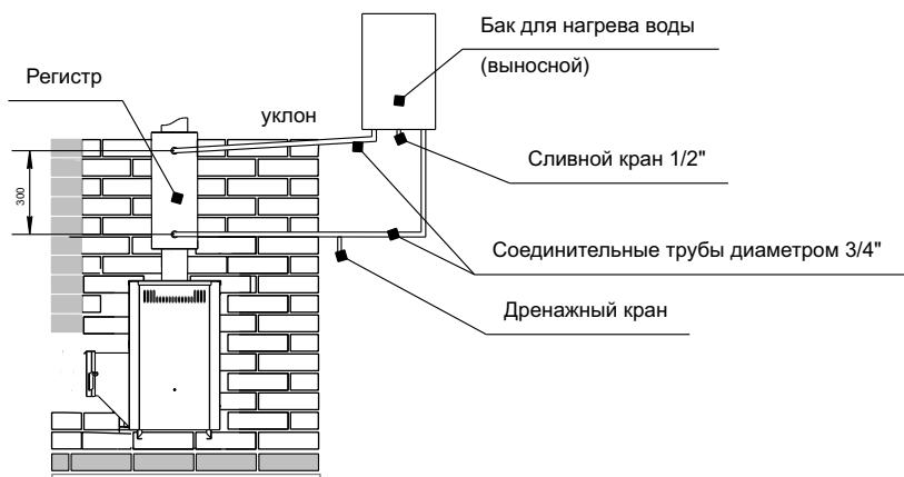
Рис. 2. Печь «ТАЙГИНКА» с дистанционным нагревом воды
