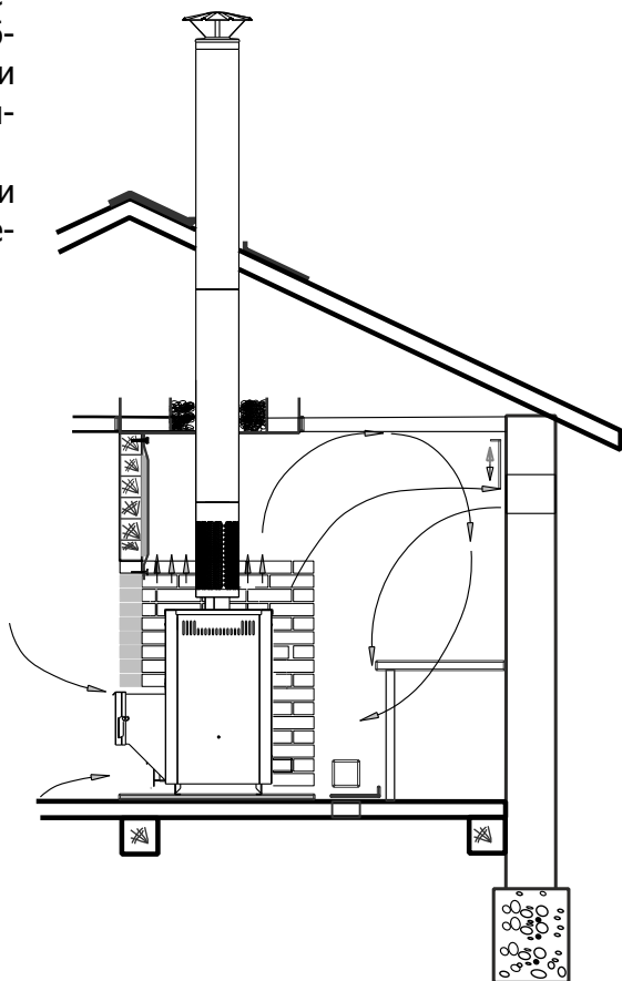
Рис. 4. Схема воздухообмена в парилке
